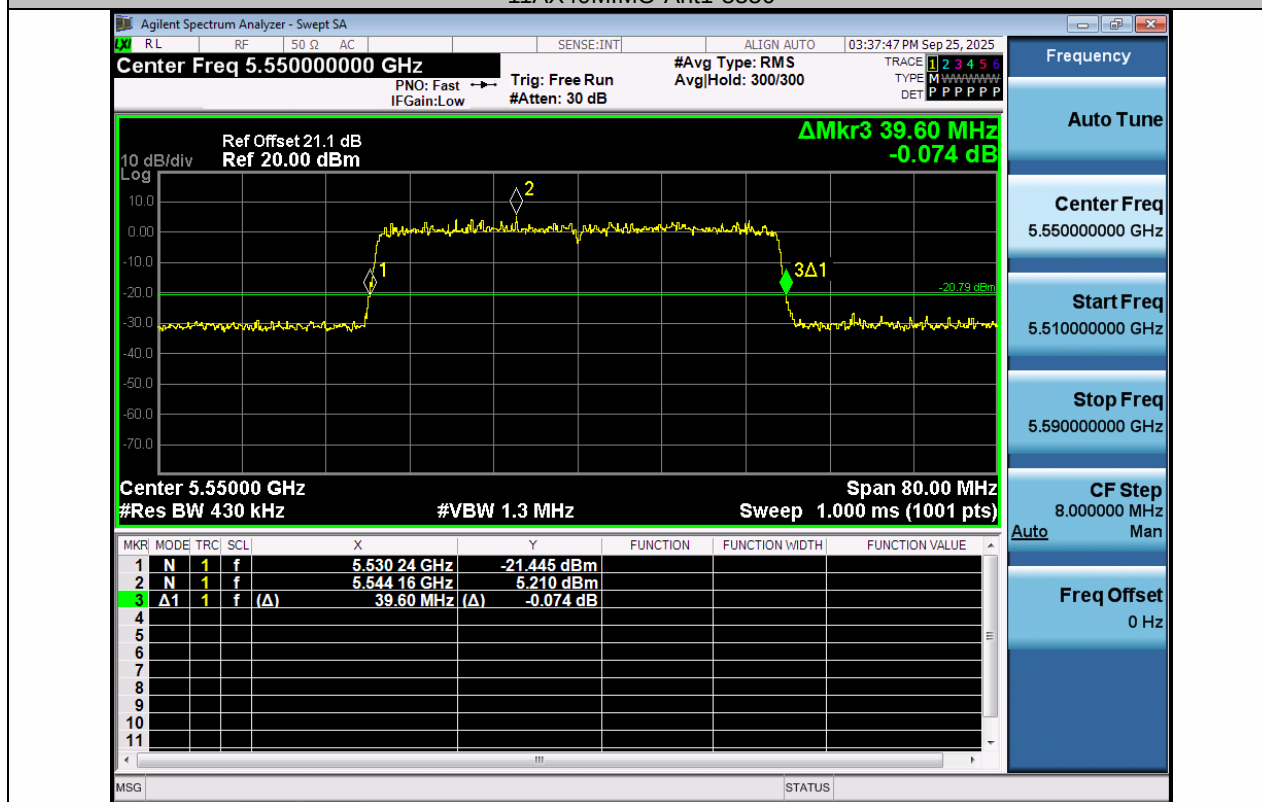
11AX40MIMO-Ant2-5550
