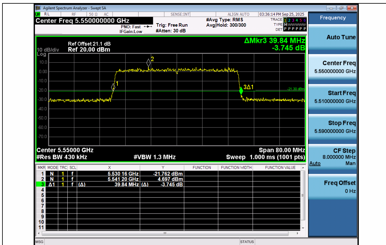
11AX40MIMO-Ant1-5550
