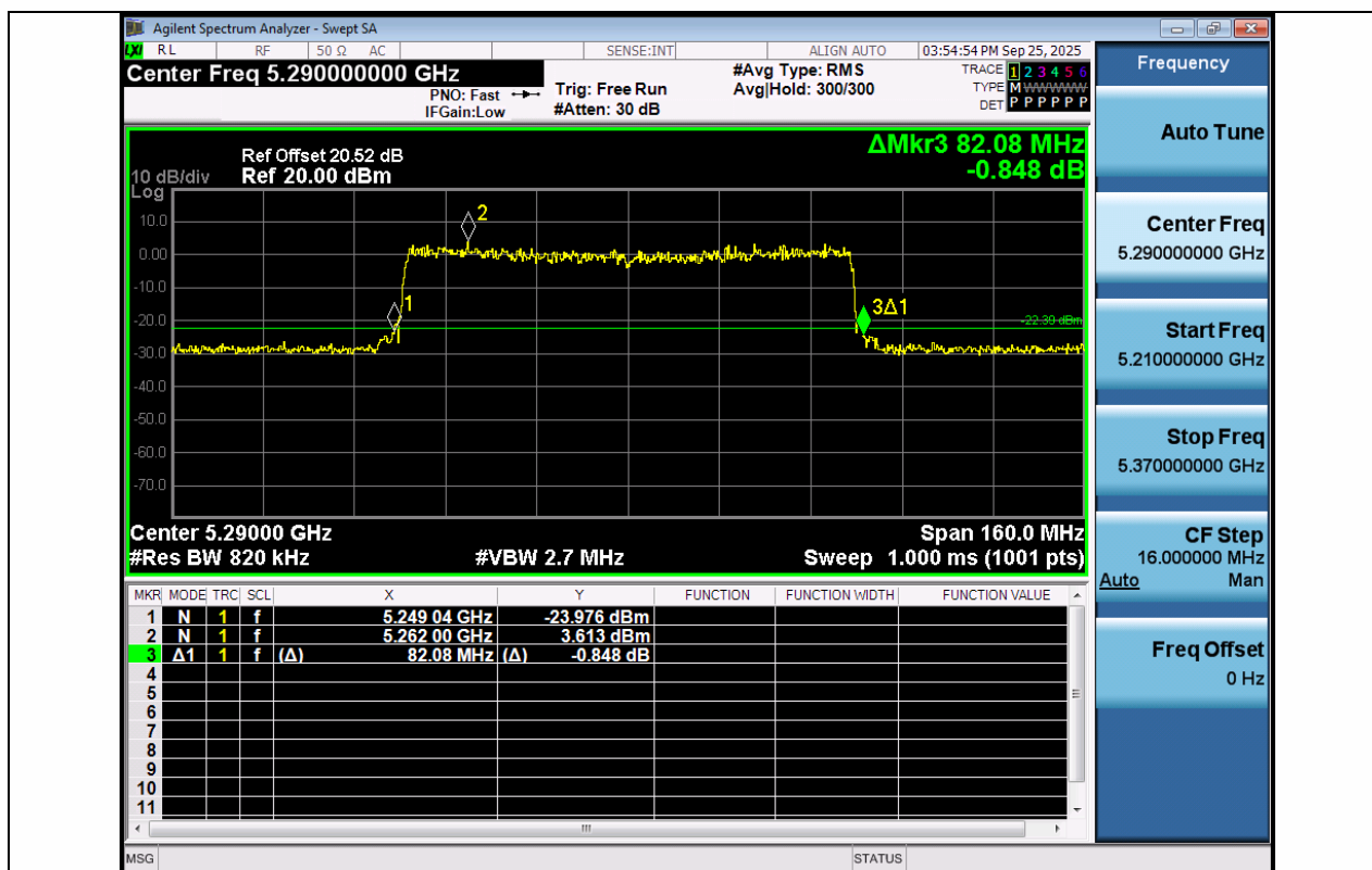
11AX80MIMO-Ant1-5290
