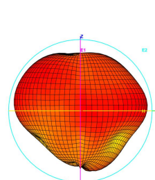
Total_3D_E2_5.85GHz
