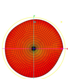
Total_3D_H_5.85GHz
