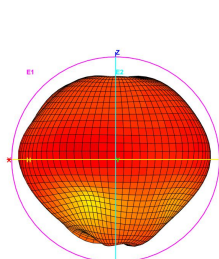
Total_3D_E1_5.85GHz
