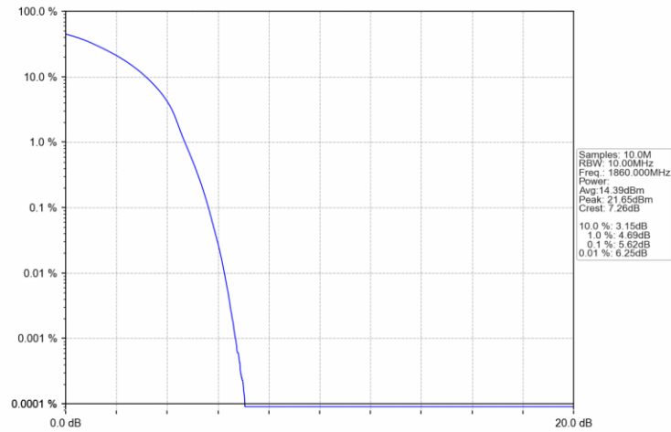
Band2 20MHz QPSK LCH 1860MHz RB 100 0 NTNV
