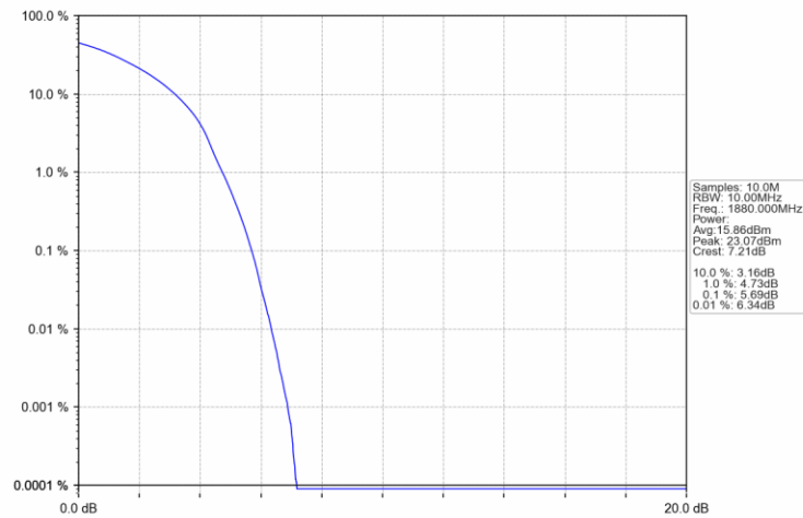
Band2 20MHz QPSK MCH 1880MHz RB 100 0 NTNV
