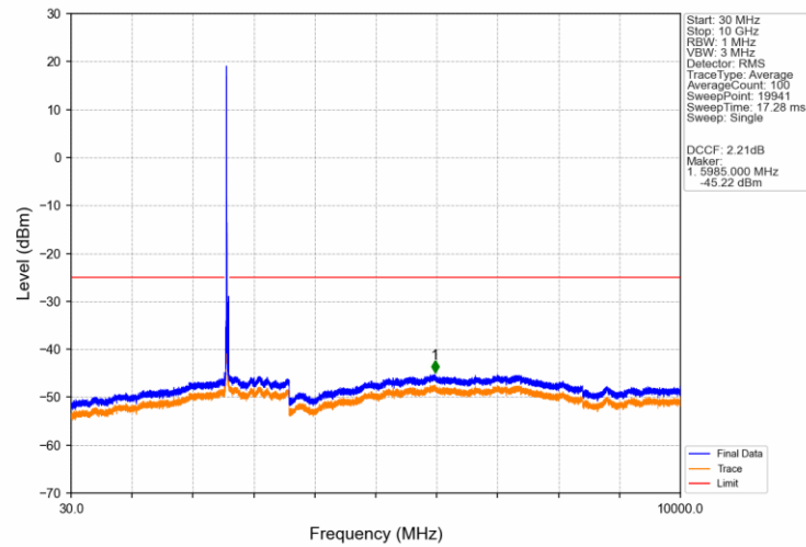
Band38 20MHz 16QAM LCH 2580MHz RB 1 0 NTNV
