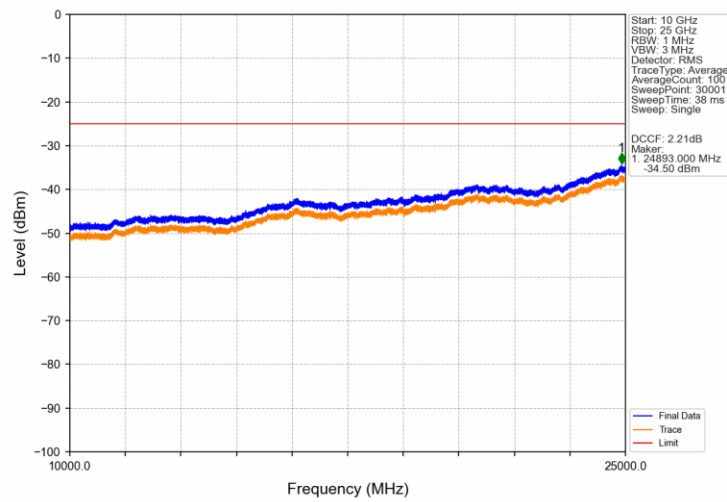
Band38 20MHz 16QAM LCH 2580MHz RB 1 0 NTNV
