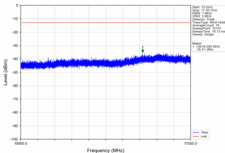
Band4_10MHz_QPSK_HCH_1750MHz_RB_1_49_NTNV
