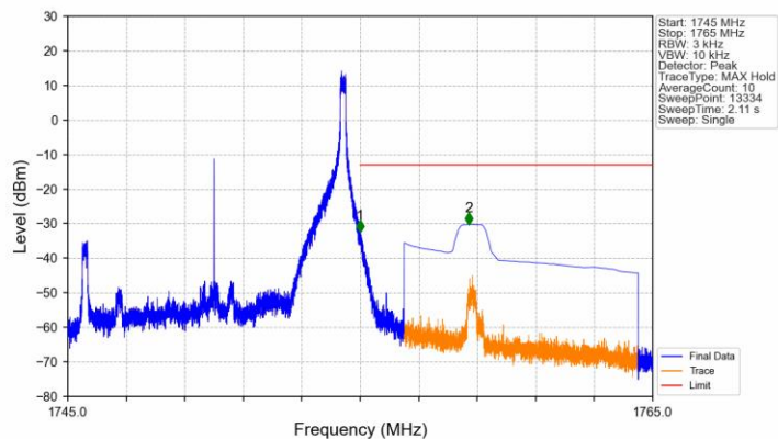
Band4_10MHz_QPSK_HCH_1750MHz_RB_1_49_NTNV
