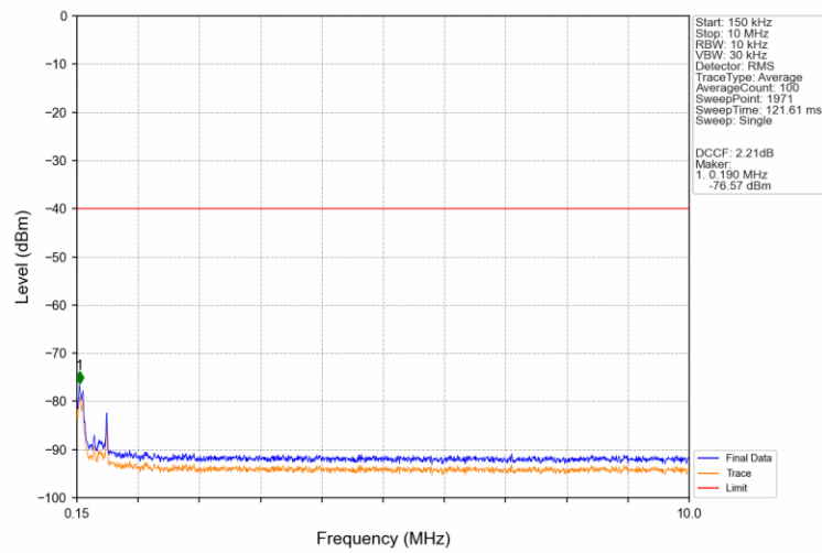
Band40b_10MHz_16QAM_LCH_2355MHz_RB_1_0_NTNV
