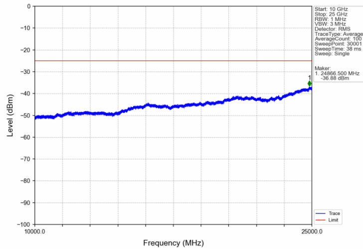
Band7 10MHz 16QAM MCH 2535MHz RB 1 0 NTNV
