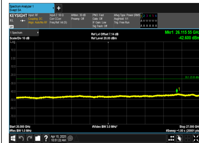
Band41-15MHz-QPSK-39725-1RB#0-20000~27000-PASS
