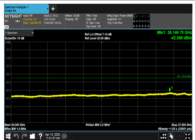
Band41-15MHz-16QAM-41515-1RB#0-20000~27000-PASS
