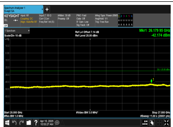
Band41-15MHz-QPSK-39725-1RB#74-20000~27000-PASS
