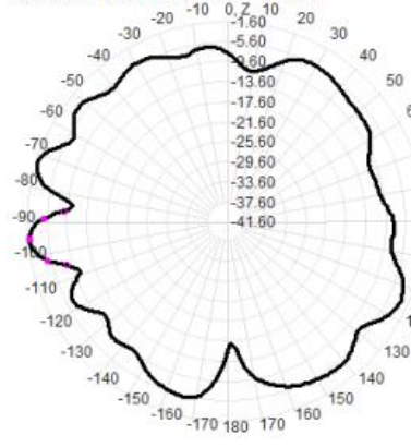
5850.0MHz Total(E1-XZ), Max=-1.92dBi
