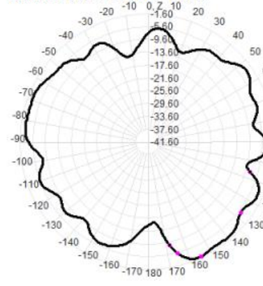
5850.0MHz Total(E2-YZ), Max=-2.28dBi
