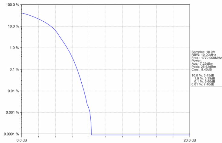
Band66 20MHz 16QAM HCH 1770MHz RB 100 0 NTNV
