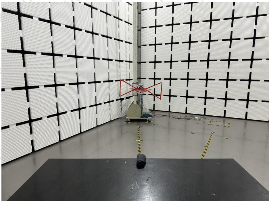
30MHz-1000MHz
