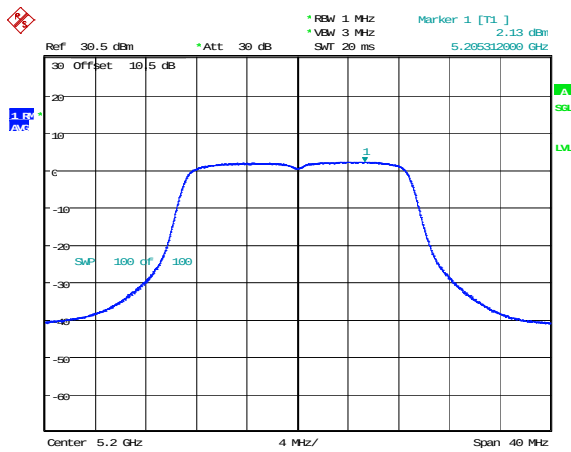
802.11n20_5200MHz_Chain 1
