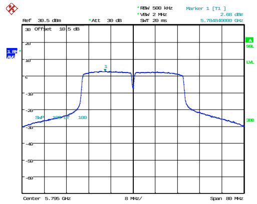
802.11n40_5795MHz_Chain 1
