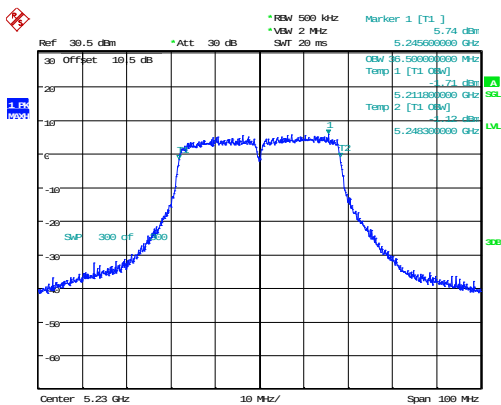
802.11n40_5230MHz_Chain 0
