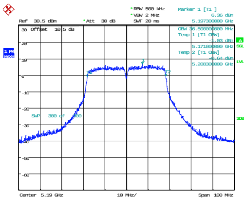
802.11n40_5190MHz_Chain 0
