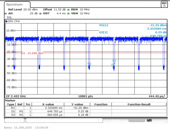
IEEE 802.11n_40MHz_Channel 9
