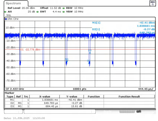
IEEE 802.11n_40MHz_Channel 3
