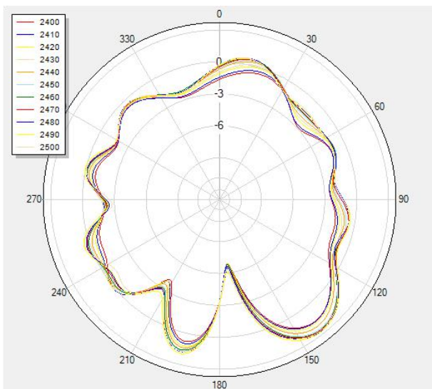
V Phi=0
