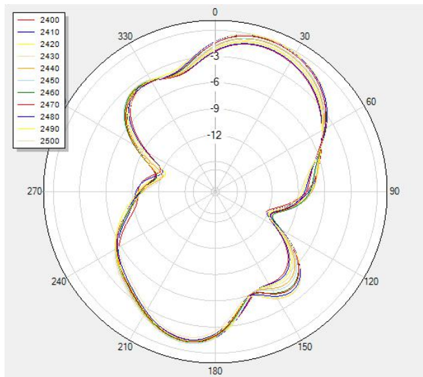
H Theta=90
