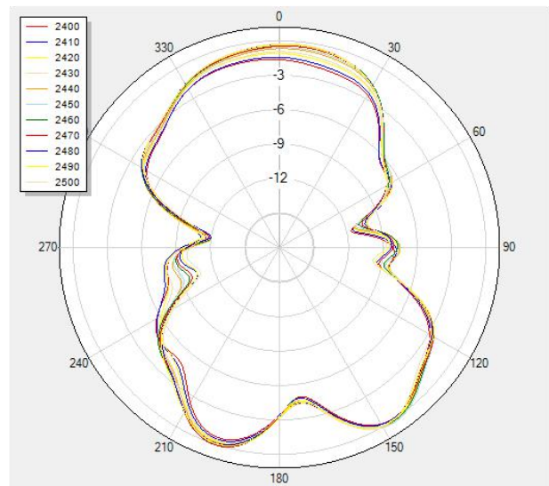
V Phi=90
