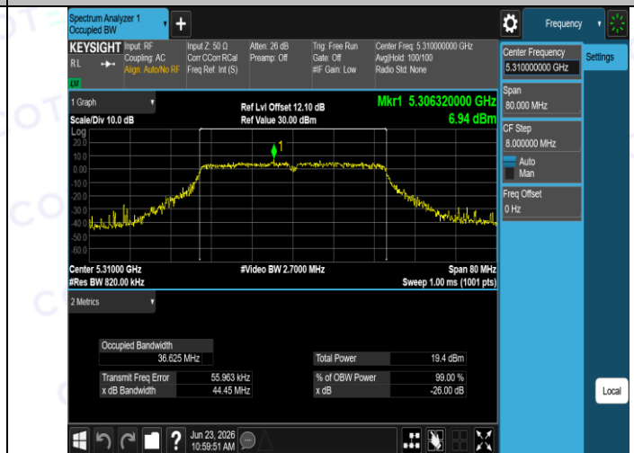
11N40SISO-Ant1-5310
