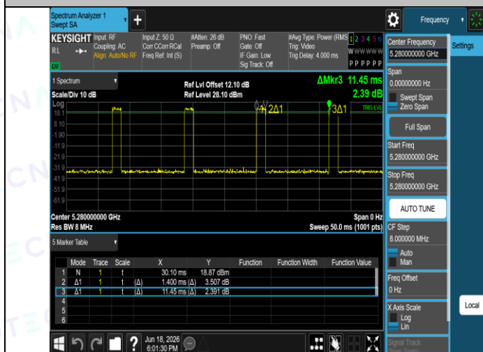
NTNV-11A-Ant1-5280
