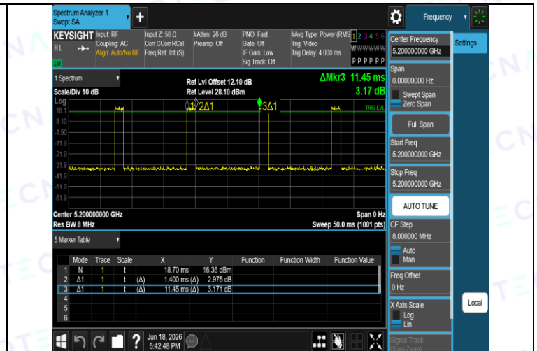
NTNV-11A-Ant1-5200
