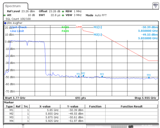
11N40SISO-Ant1-5755-PASS
