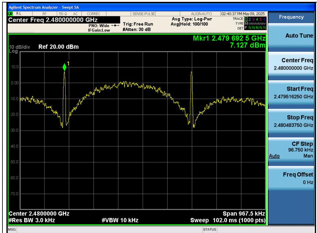
Test_Graph_LE500K_ANT1_2480_500Kbps_PSD
