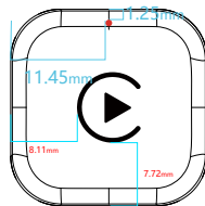
顶面
