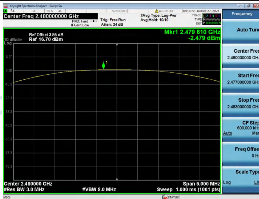
Peak_Output_Power_NVNT_ANT1_1Mbps_2480
