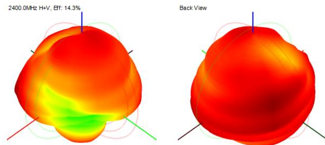
2400.0MHz Total(E1), Max=-5.33dBi
