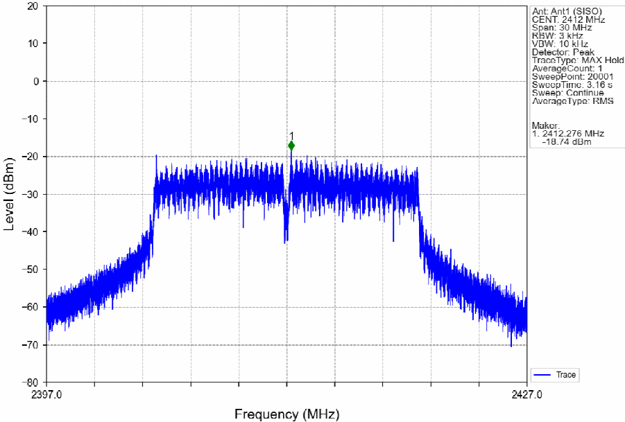
802.11g_LCH_2412MHz_Ant1 (SISO)_NTNV
