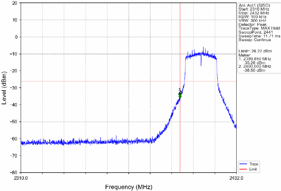
802.11n(HT20)_LCH_2412MHz_Ant1 (SISO)_NTNV
