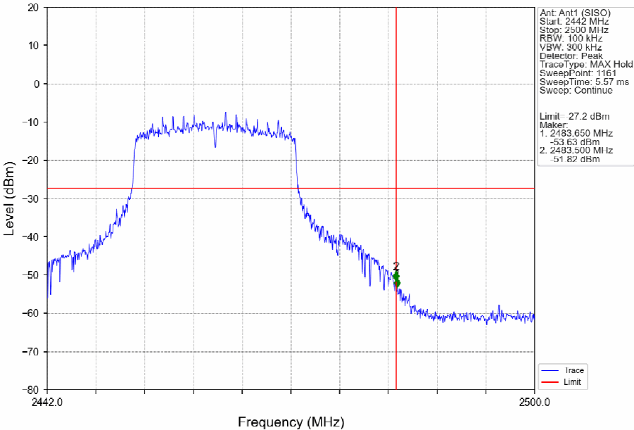
802.11ax(HEW20)_HCH_2462MHz_SU_/_Ant1 (SISO)_NTNV
