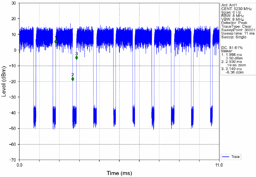
802.11n(HT40) HCH_5230MHz_Ant1_NTNV
