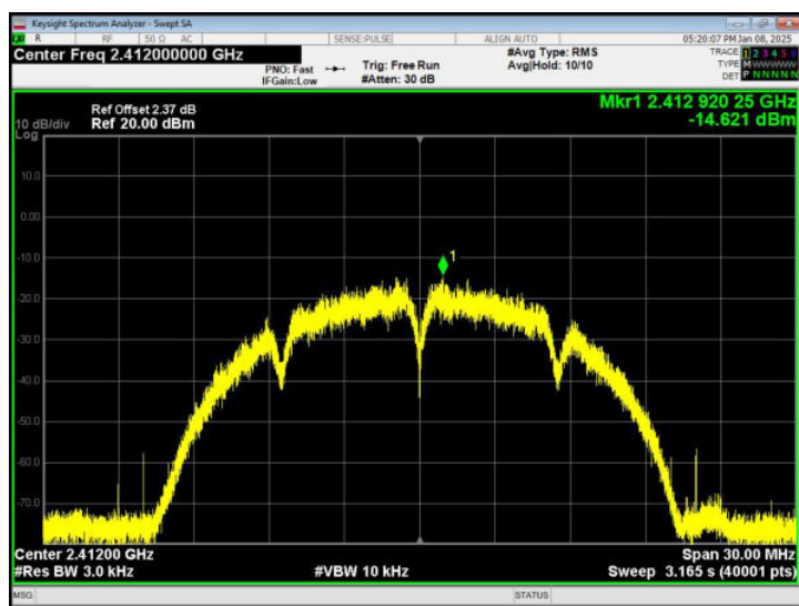
802.11b - CH01
