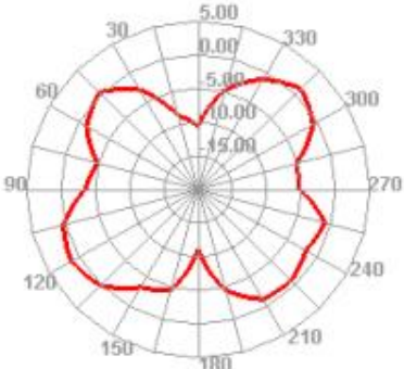
2450.000MHz E1
