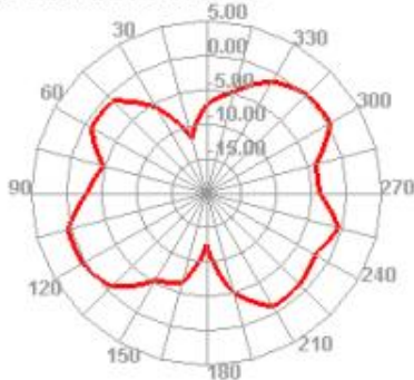
2400.000MHz E1
