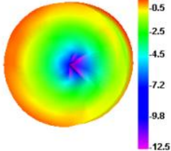
2400.000MHz
