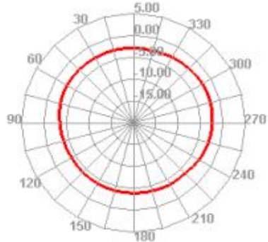
2400.000MHz H
