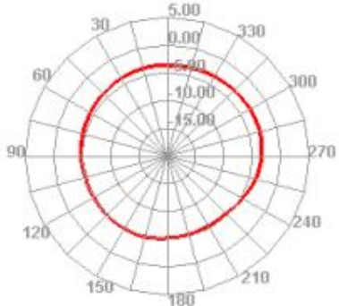
2450.000MHz H
