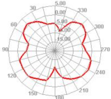
2450.000MHz E2
