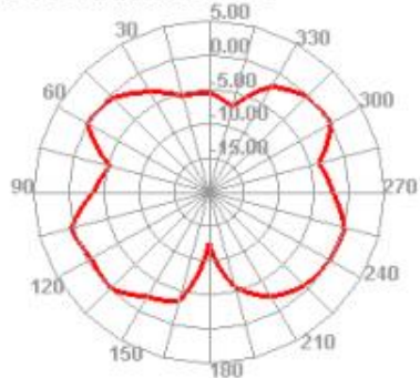
2400.000MHz E2
