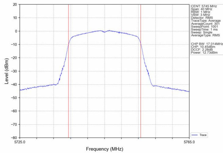
802.11a_LCH_5745MHz_Ant2_NTNV
