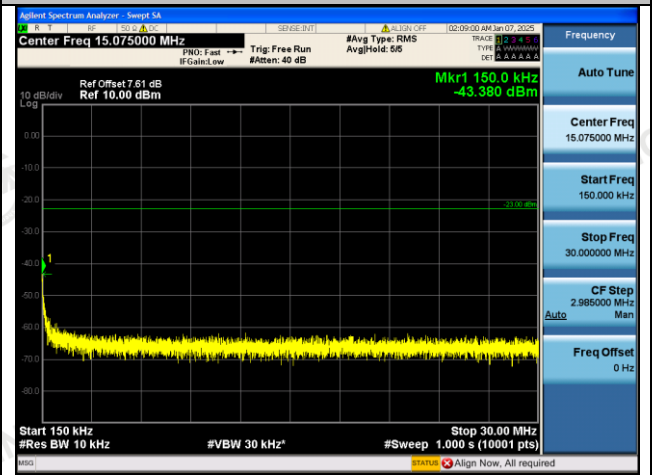
GSM850-190-5-0.15~30MHz-PASS
