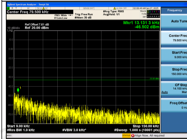
GSM850-190-5-0.009~0.15MHz-PASS
