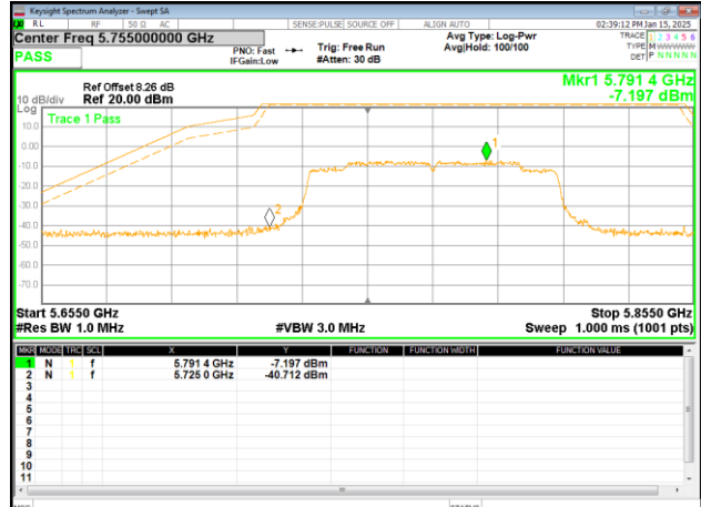
(802.11ax80) Band Edge
