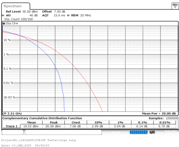
20MHz_Middle_QPSK_100@0
