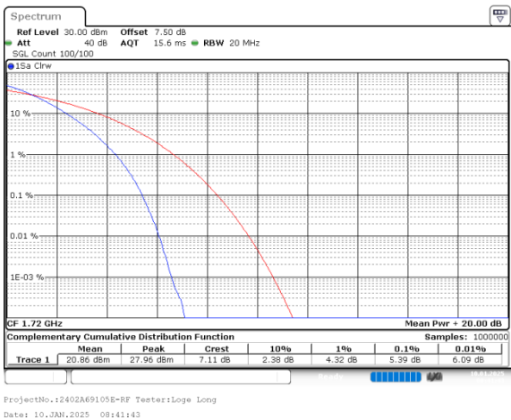
20MHz_Low_16QAM_25@0
