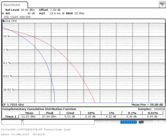
20MHz_Middle_QPSK_100@0
