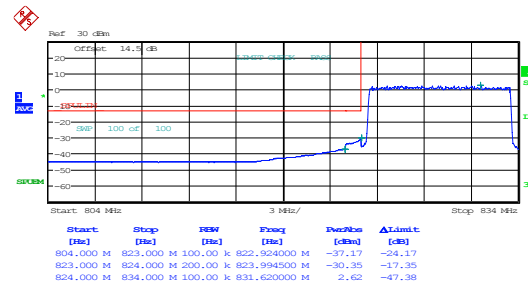
10MHz_Low_QPSK_50@0
