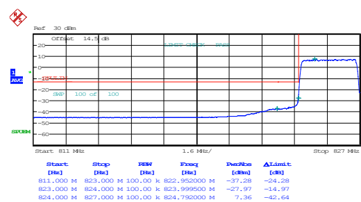
3MHz_Low_16QAM_15@0
