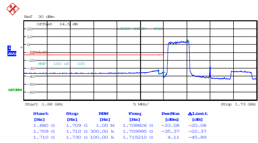
20MHz_Low_16QAM_25@0
