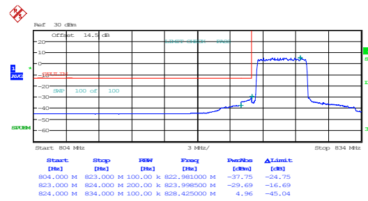
10MHz_Low_16QAM_25@0
