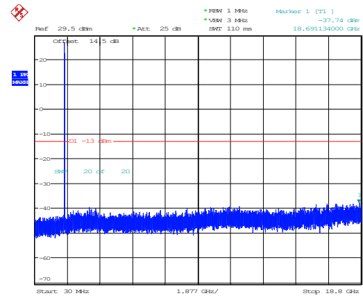
5MHz_Middle_QPSK_1@0(30MHz~18.8GHz)
