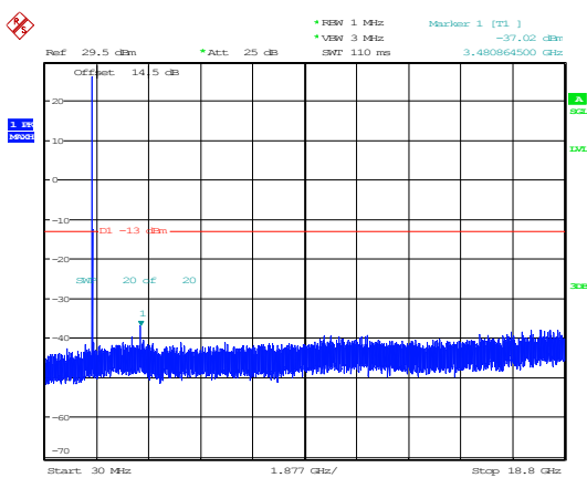
10MHz_Middle_QPSK_1@0(30MHz~18.8GHz)
