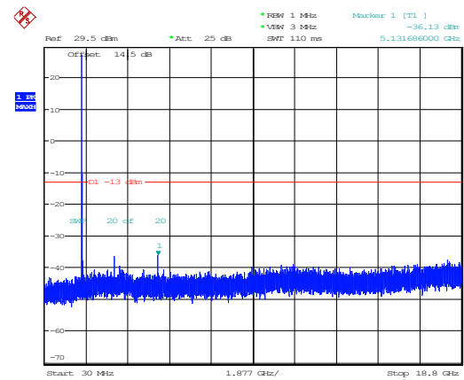
10MHz_Low_QPSK_1@0(30MHz~18.8GHz)
