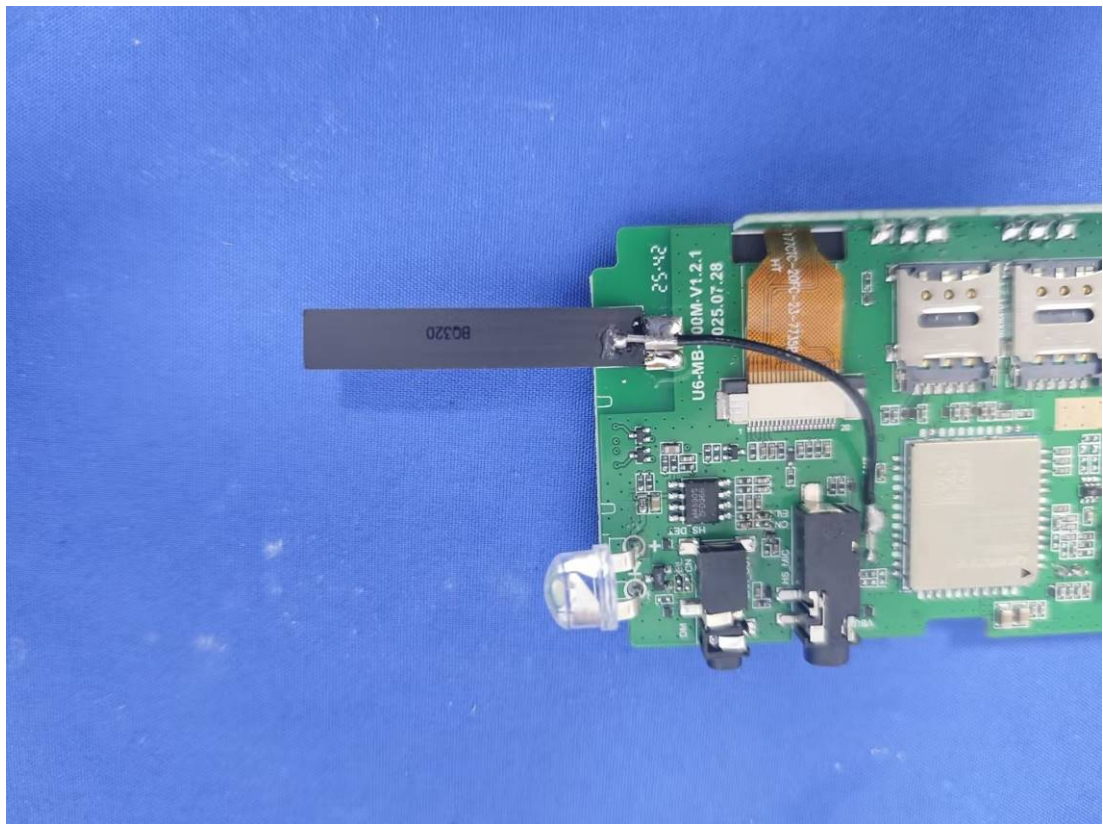
LTE Antenna
