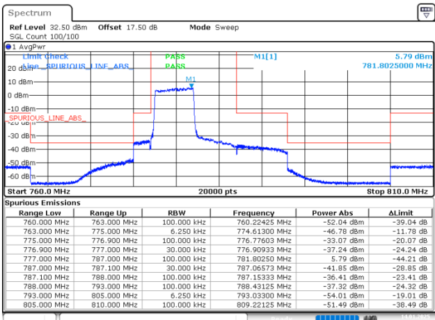
10MHz_Middle_16QAM_25@0
