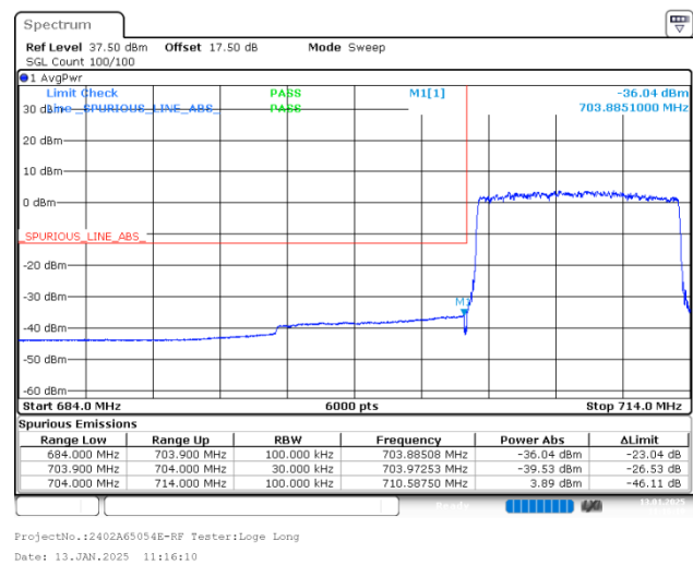
10MHz_Low_QPSK_50@0
