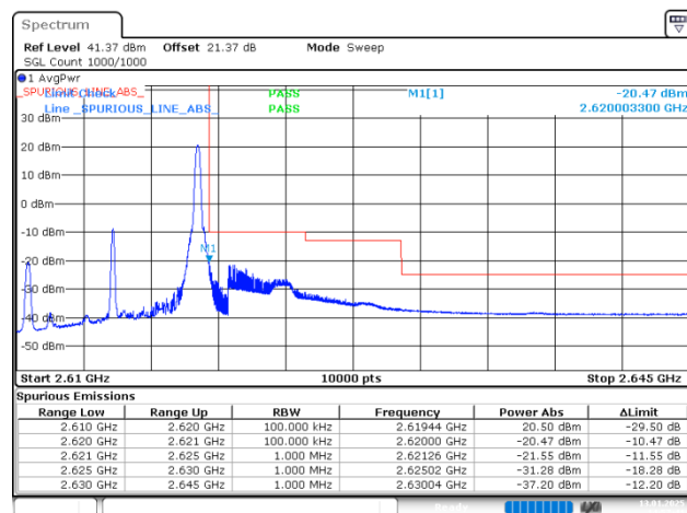
10MHz High QPSK 1@49
