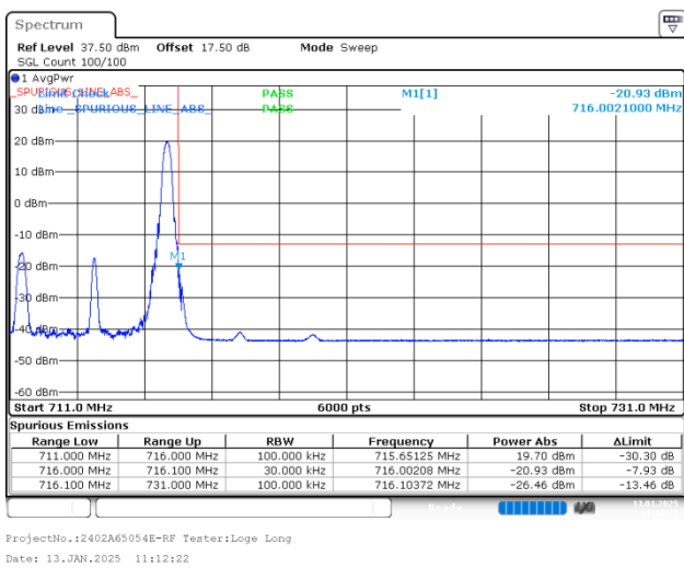
10MHz_Low_QPSK_1@0
