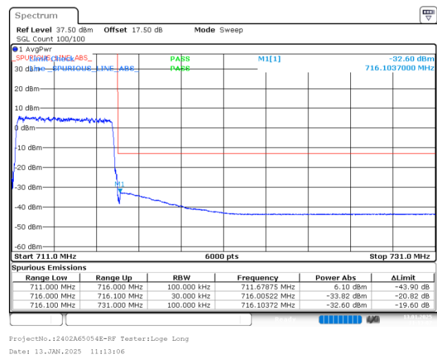
10MHz_Low_QPSK_50@0
