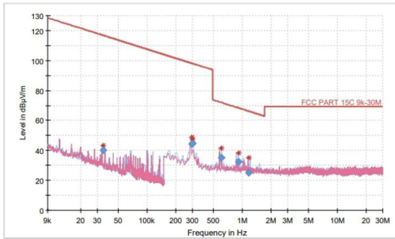
CH 39(High)
