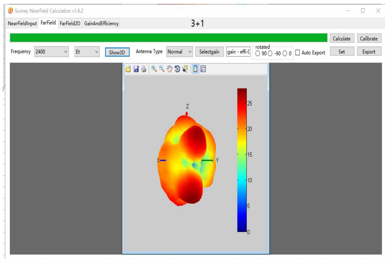
BT 天线苹果图 (BT antenna apple diagr)
