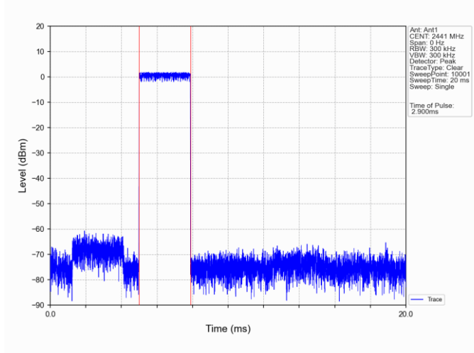
GFSK_DH5_HOPP_Ant1_NTNV
