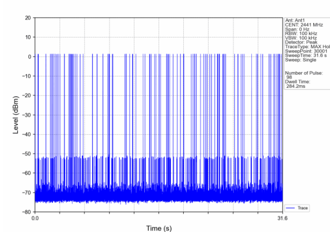
GFSK_DH5_HOPP_Ant1_NTNV
