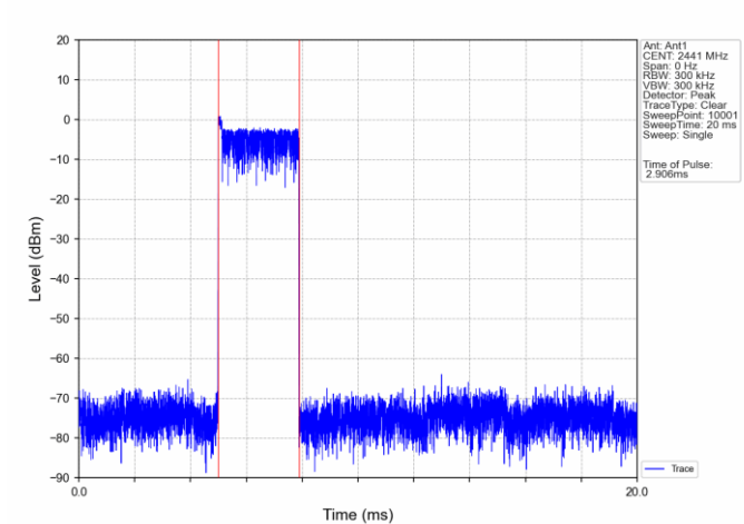
Pi/4DQPSK_2DH5_HOPP_Ant1_NTNV
