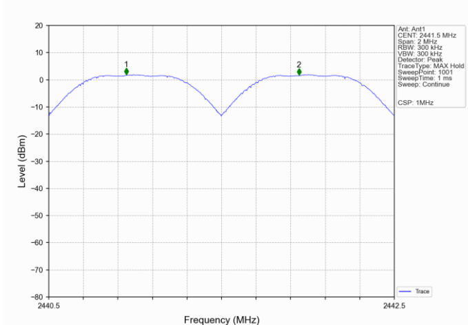
GFSK_DH5_HOPP_Ant1_NTNV
