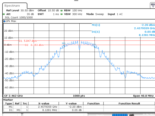
802.11b_2462MHz
