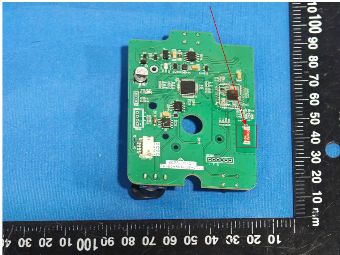
Bluetooth&Wifi Antenna
