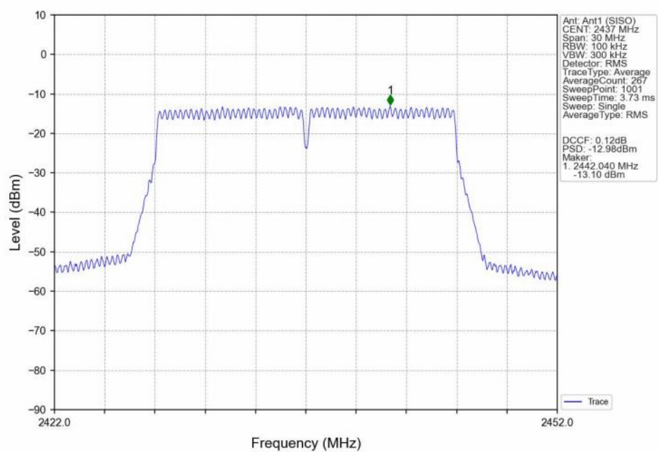
802.11ax(HEW20)_MCH_2437MHz_SU_/_Ant1 (SISO)_NTNV
