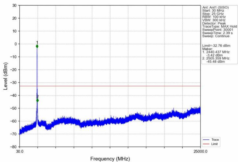
802.11ax(HEW40)_MCH_2437MHz_SU_/_Ant1 (SISO)_NTNV
