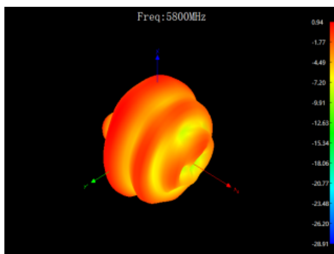
5800MHZ
