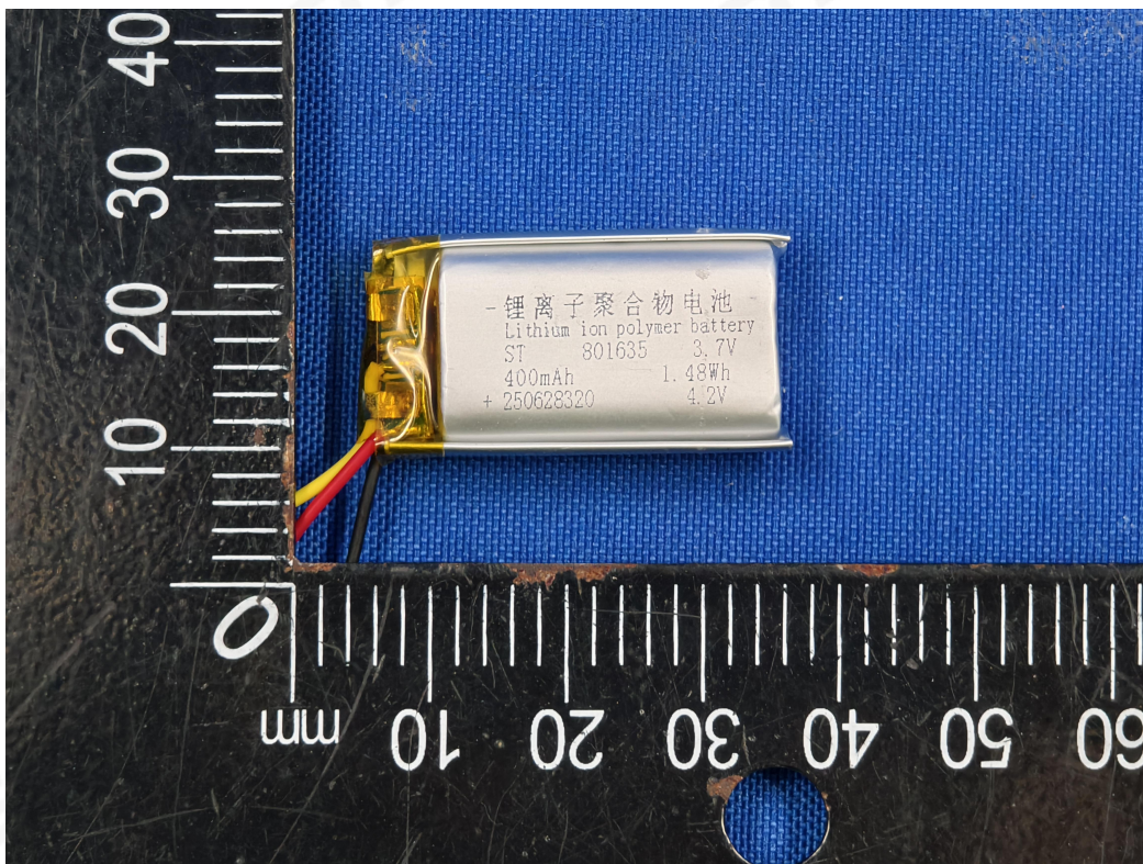
Photo 8 (电池照有误)
