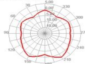
2500.000MHz E1
