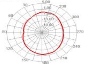
2500.000MHz H
