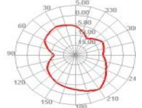
2400.000MHz E2
