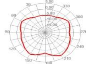
2400.000MHz E1
