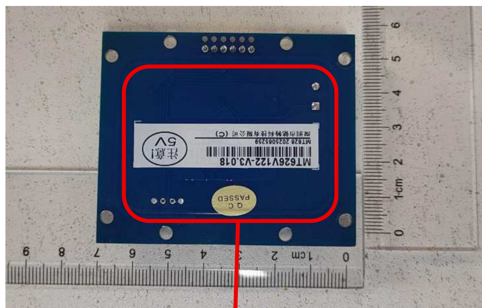
Antenna
