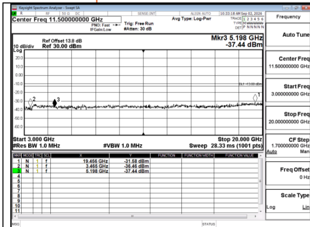
HSPA_HSPA_B4_Mid CH1413-1732.6_MidCH1413-1732.6
