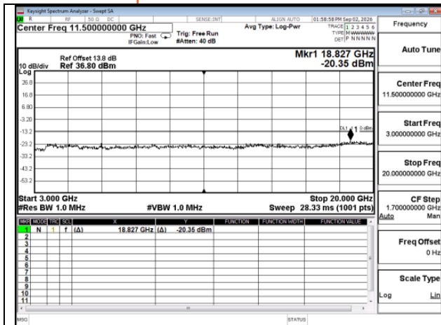
GPRS_GPRS_1900MHz_Mid CH661-1880_MidCH661-1880
