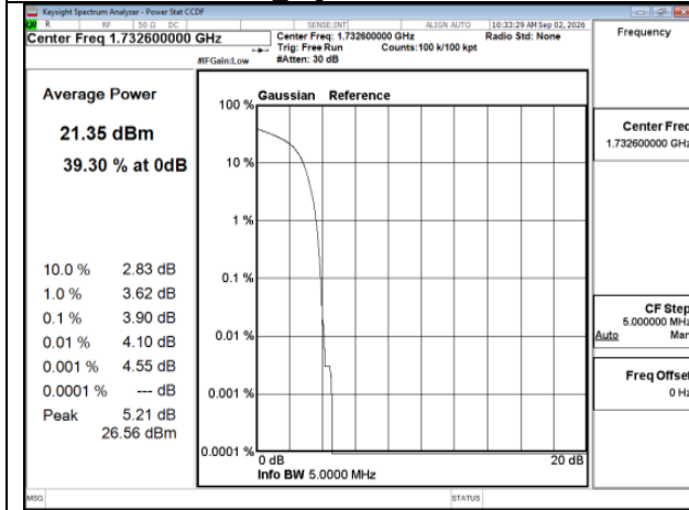
HSPA_B4_Mid CH1413-1732.6_MidCH1413-1732.6
