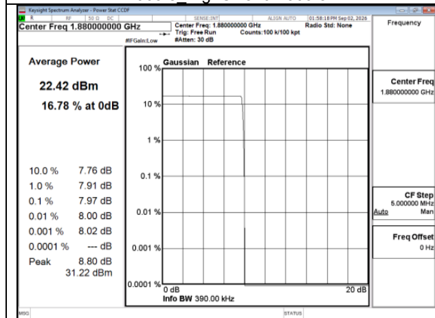
GPRS_GPRS_1900MHz_Mid CH661-1880_MidCH661-1880
