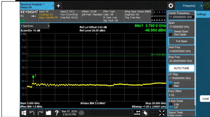
GPRS1900-661-0-3000~20000MHz-PASS
