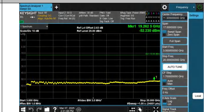
GPRS1900-512-0-3000~20000MHz-PASS
