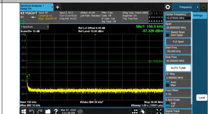
GPRS1900-661-0-0.15~30MHz-PASS
