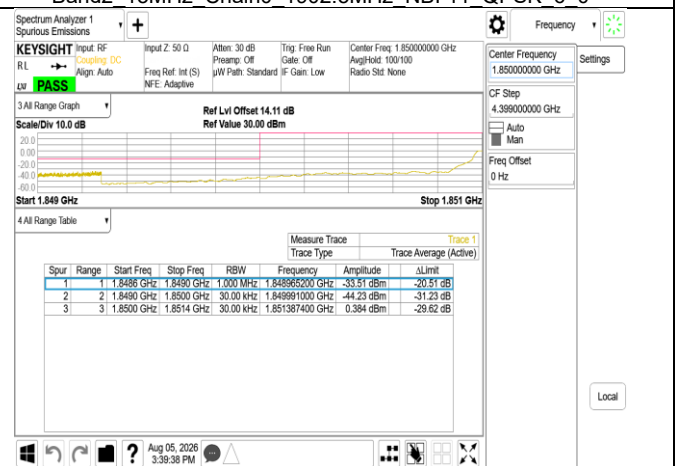
Band2 20MHz Chain0 1860MHz NBI 0 QPSK 6 0
