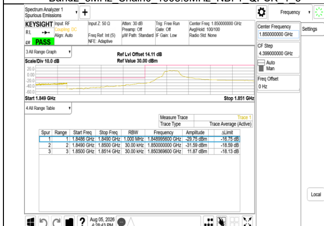
Band2 5MHz Chain0 1852.5MHz NBI 0 QPSK 1 0
