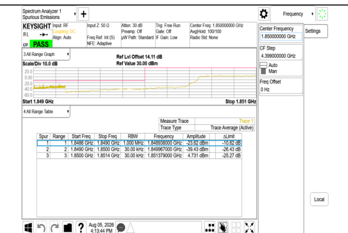
Band2 10MHz Chain0 1855MHz NBI 0 QPSK 6 0
