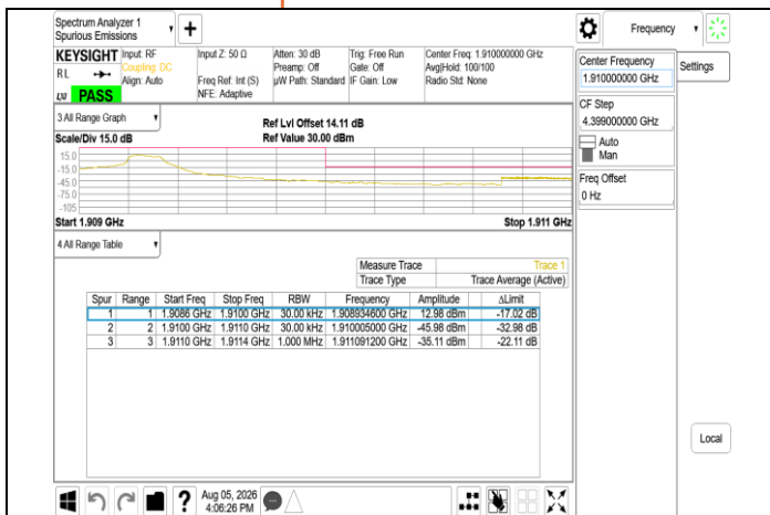
Band2 15MHz Chain0 1902.5MHz NBI 11 QPSK 1 5
