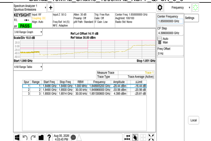
Band2 15MHz Chain0 1857.5MHz NBI 0 QPSK 6 0
