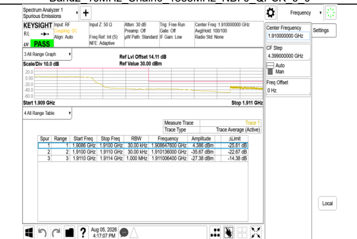
Band2 10MHz Chain0 1905MHz NBI 7 QPSK 6 0
