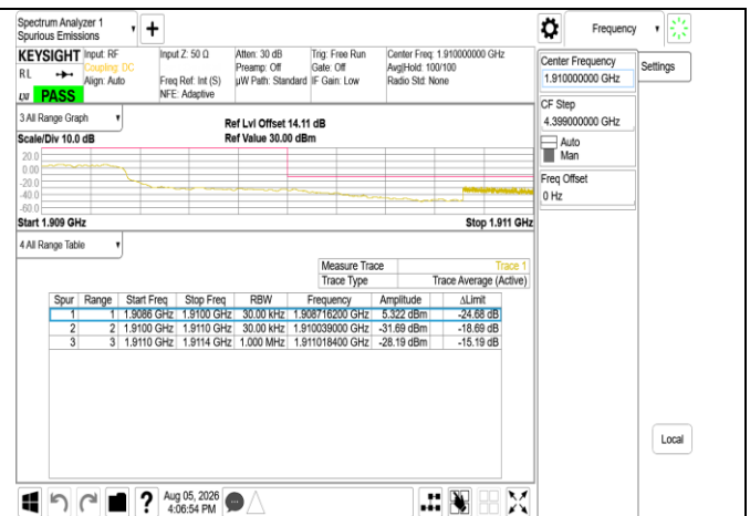
Band2 15MHz Chain0 1902.5MHz NBI 11 QPSK 6 0
