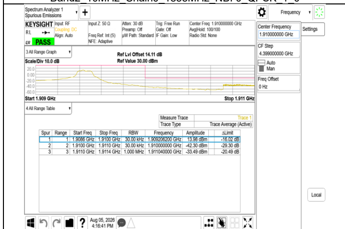
Band2 10MHz Chain0 1905MHz NBI 7 QPSK 1 5
