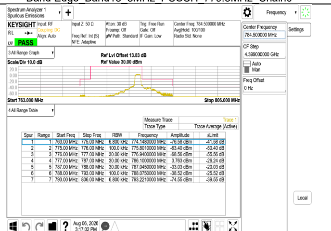
Band Edge Band13 5MHz PUSCH 784.5MHz Chain0
