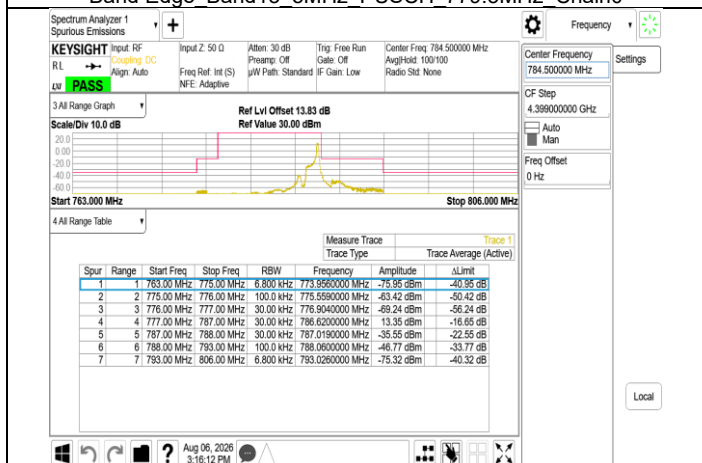
Band Edge Band13 5MHz PUSCH 784.5MHz Chain0
