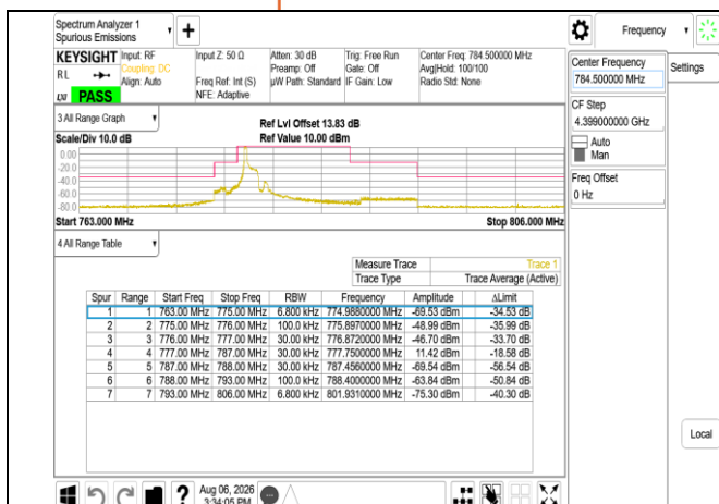
Band Edge Band13 10MHz PUSCH 782MHz Chain0
